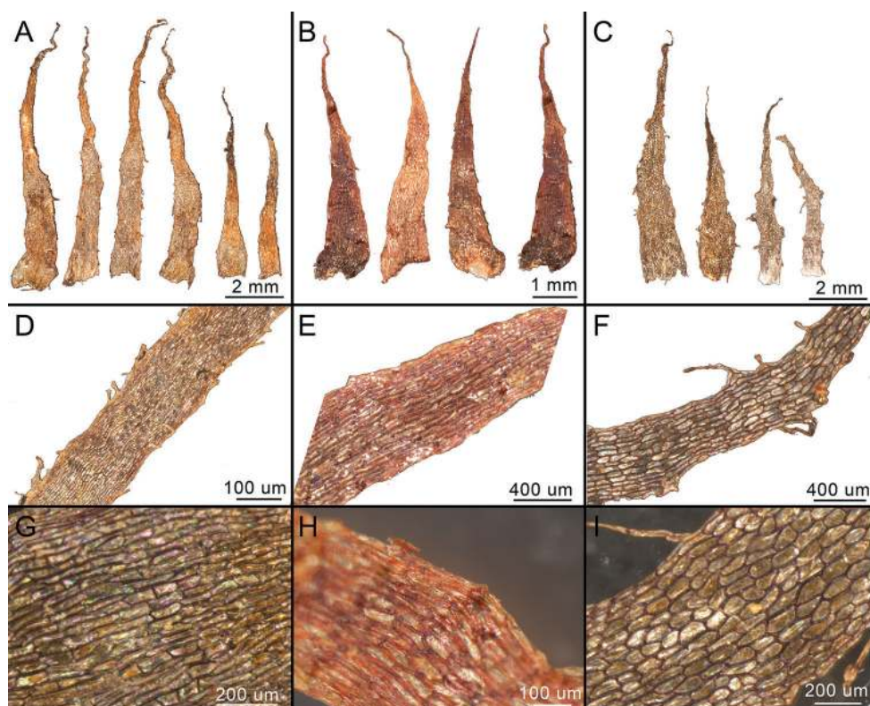
Figure 2. Scales of A. alatum , A. subcrenatum and A. wrightii . A, D, G A. wrightii B, E, H A. subcrenatum C, F, I A. alatum .
