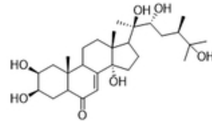
Makisterone-A (4)
