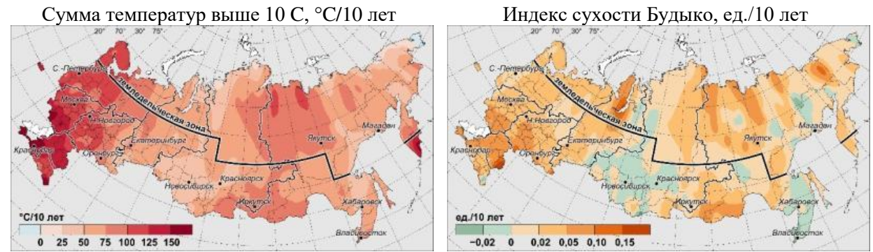
Рисунок 8.3 – Скорость изменения (линейный тренд) суммы температур выше 10°C (°C/10 лет) и индекса сухости М.И. Будыко (ед./10 лет) за период 1976-2024 гг.
