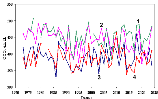
Рисунок 18.2 – Межгодовой ход средних за март значений ОСО на станциях: 1 – Нагаево (Магадан) (60° с.ш., 151° в.д.), 2 – Якутск (62° с.ш., 130° в.д.), 3 – С.-Петербург (60° с.ш., 30° в.д.) и 4 – Екатеринбург (57° с.ш., 61° в.д.)
