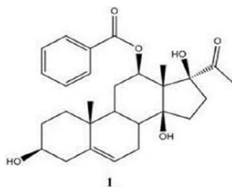
Calotropone
