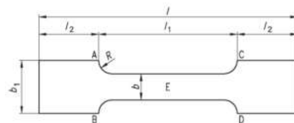
Figura 1. Diseño de la Probeta
