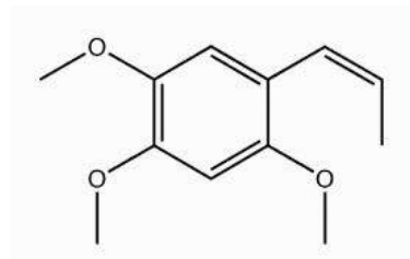
Gambar 5.6 Struktur Kimia Asarone
