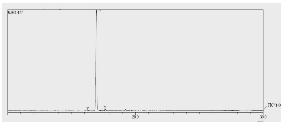
Gambar 5.5 Kromatografi Gas Isolat F14
