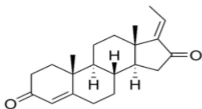
Fig. 1. Guggulsterone
