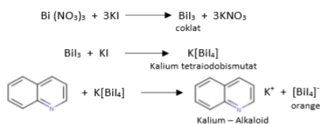
Gambar 1 Reaksi Uji Dragendroff
