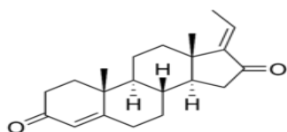
Fig. 1. Guggulsterone
