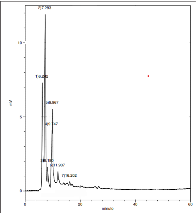
Figure 1. EESD chromatogram.
