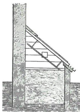
En af de Lindegaardske vinbakker tegnet i snit. Vinrankerne føres gennem det firkantede hul i gavlen ind i huset; varmen leveres dels af solen dels af det tykke lag staldgødning der, som det ses, fylder ca. halvdelen af rummet ud.
