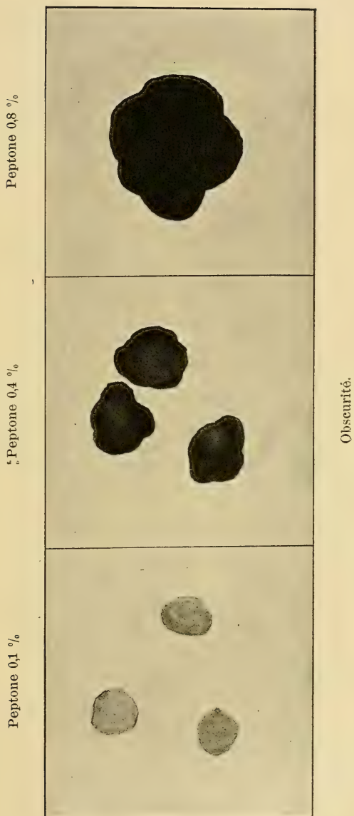
Fig. 1. — CHLORELLA PROTOTHECOIDES
