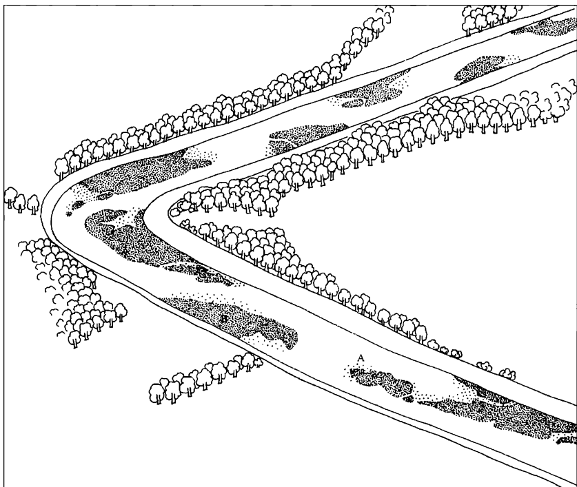
Abb. 1: Schematische Darstellung der Schotterbanktypen im Fürstentum Liechtenstein. A = isolierte Inseln, B = Schotterbänke mit Uferkontakt.
