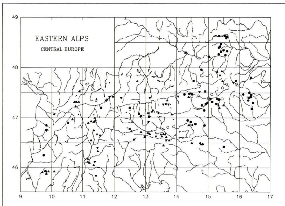
Abbildung 1: Biotope auf Schwermetallstandorten im Ostalpenraum (vgl. Tab. 1): Galmei (▲); Kupfer (▼); Serpentin/Chrom (●); Magnesit (○); Arsen/ Antimon (◆); Andere (■). Mielichhoferia -Standorte nach verschiedenen Quellen, v.a. GRIMS (schriftl. Mitt.): •.
