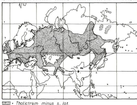
Abb.4: Verbreitung von Thalictrum minus s.lat. (nach MJW 1965)
