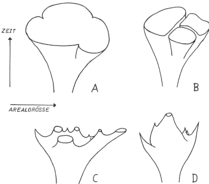
Abb.14: Veränderungen der Areale in der Zeit, schematisch (in Anlehnung an EHRENDORFER 1983)
