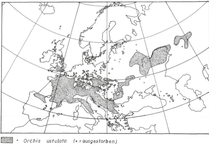
Abb.13: Verbreitung von Orchis ustulata - verbesserte Karte (nach MEUSEL und KNAPP 1983)
