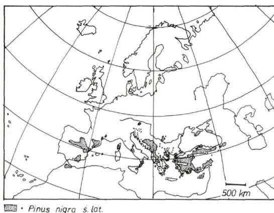
Abb.5: Verbreitung von Pinus nigra s.lat. (nach MJW 1965)
