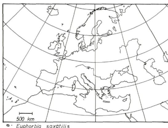
Abb.6: Verbreitung von Euphorbia saxatilis (nach MJW 1965)
