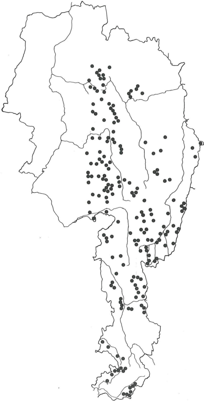
Abb. 7. Verbreitung von Silene pusilla Waldst. & Kt. in Österreich.
