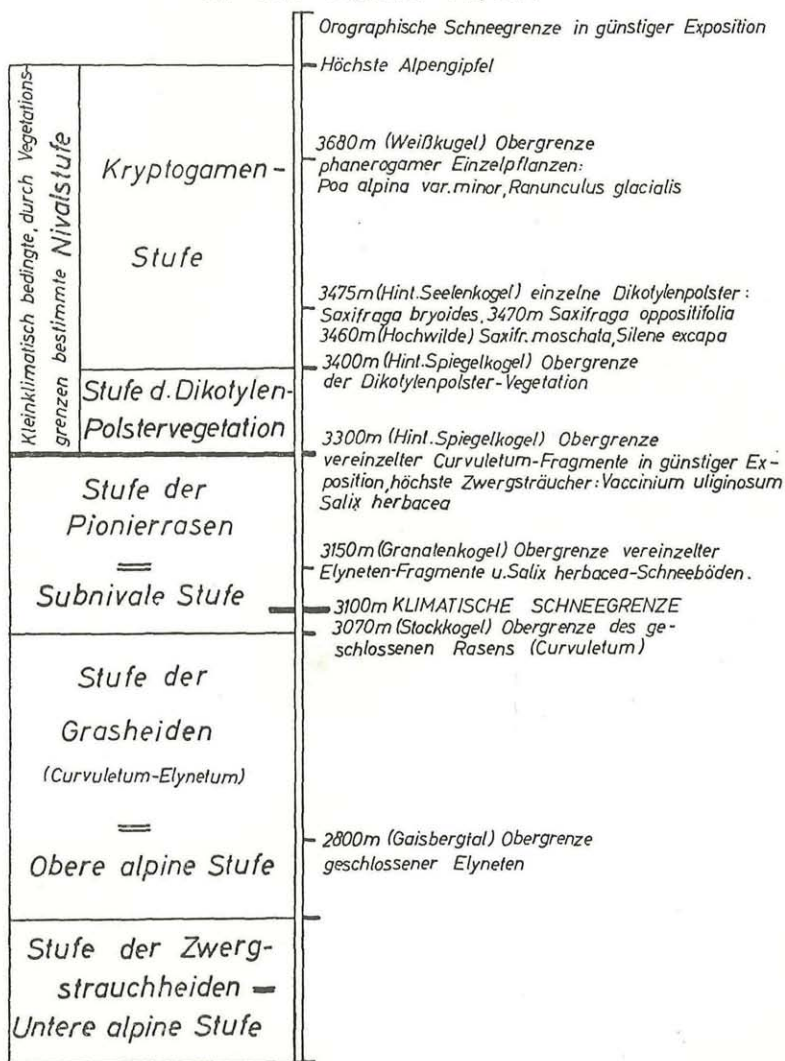
Abb. 1: Schema der vertikalen Gliederung der Vegetation in den Öztaler Alpen. (Nach REISIGL & PITSCHMANN 1958: 105).
