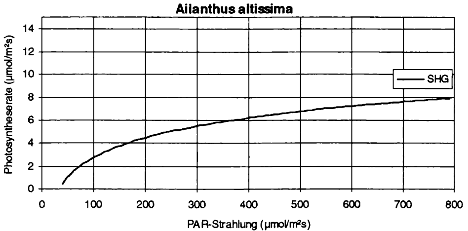
Abb. 4: Lichtsättigungskurve von Ailanthus am Standort Schlachthausgasse (= SHG; EISINGER 1996a) – Light saturation graph of Ailanthus on a near-city site
