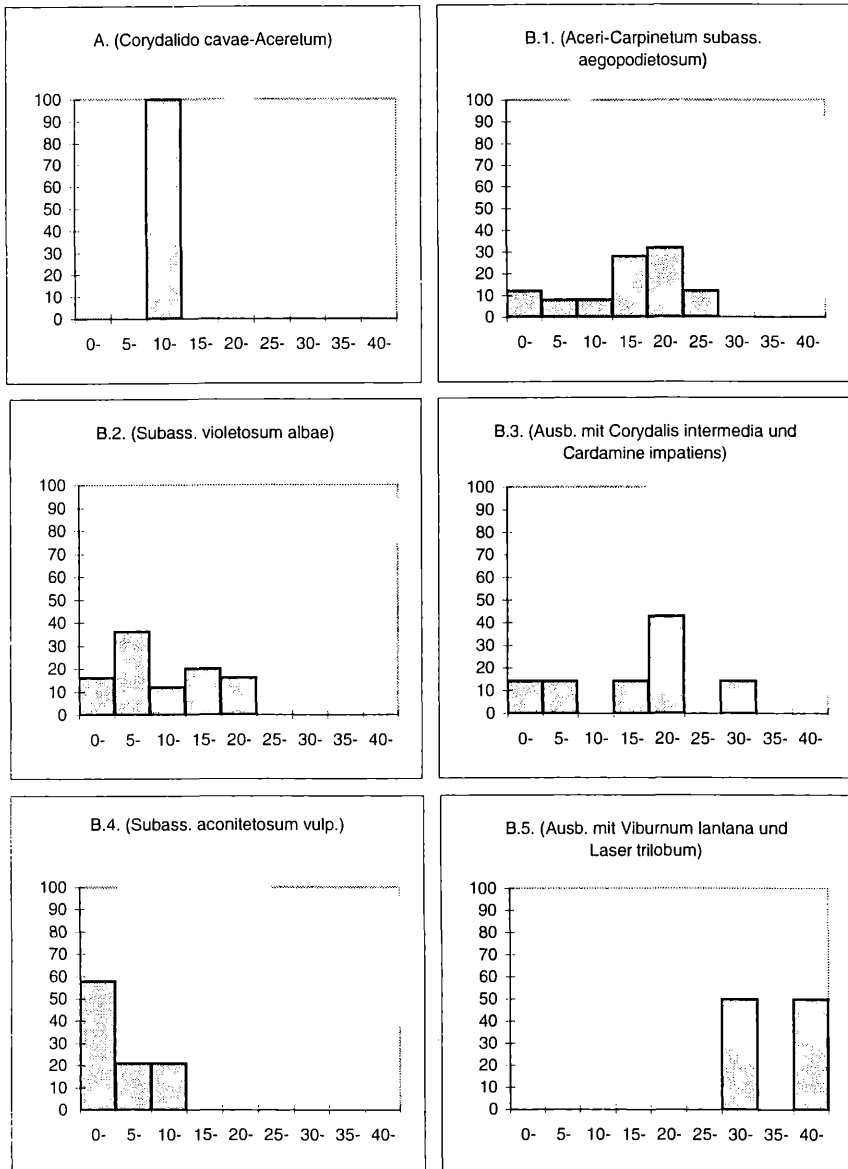
Abb. 4: Verteilung der Hangneigungen in den pflanzensoziologischen Einheiten. Horizontal: Vertikal: %. — Distribution of inclination within the phytosociological units. Horizontal: Vertikal: %.
