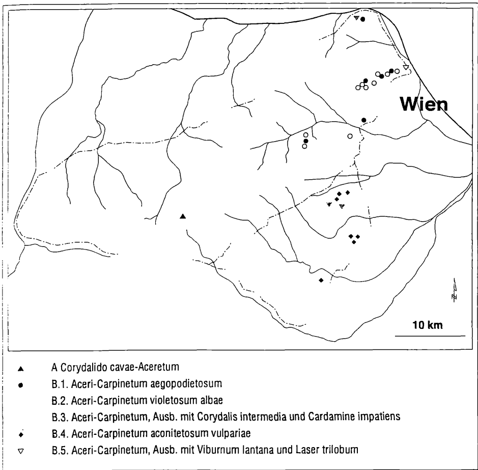
Abb. 1: Verbreitung der pflanzensoziologischen Einheiten im Wienerwald. Die durchbrochene Linie gibt die Umgrenzung von Flysch- und Kalkwienerwald wieder. — Distribution of the phytosociological units in the study area. The pierced line shows the boundary of Sandstone and Limestone Wienerwald.
