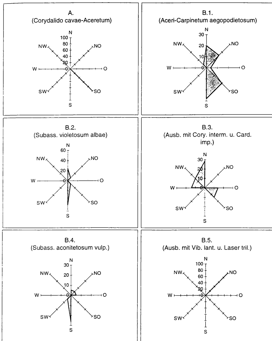
Abb. 3: Prozentuelle Verteilung der Expositionen in den pflanzensoziologischen Einheiten. — Distribution of exposition within the phytosociological units (in %).
