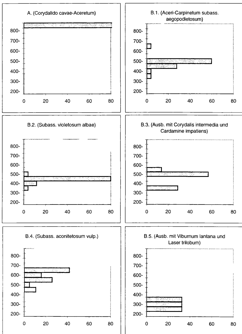
Abb. 2: Verteilung der Seehöhen in den pflanzensoziologischen Einheiten. Horizontal: %. Vertikal: m.s.m. — Distribution of altitude within the phytosociological units. Horizontal: %. Vertical: m.s.m.
