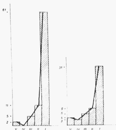
Obr. 1. — Presencí - křivky as. Carici leporinae-Agrostetum tenuis (vlevo) a as. Nardo-Juncetum squarrosi (vpravo). — Abb. 1. — Stetigkeitsdiagramm der Ass. Carici leporinae-Agrostetum tenuis (links) und der Ass. Nardo-Juncetum squarrosi (rechts).
