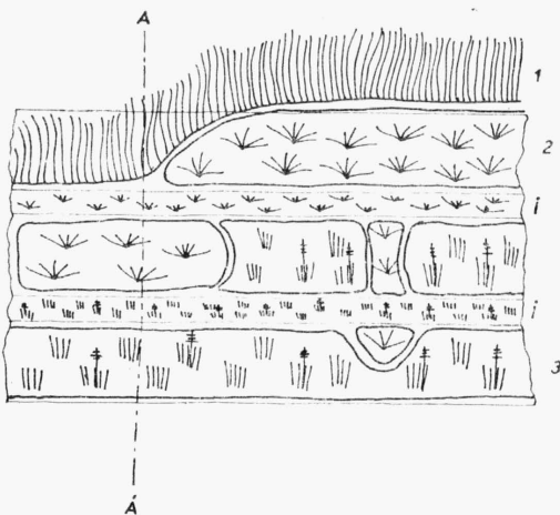
Obr. 4. — Schematický náčrt vegetace cesty na Z svahu Ještědu (Ještědské pohoří): 1 — pasekové společenstvo s Calamagrostis villosa , 2 — Nardo-Juncetum squarrosi , 3 — Carici leporinae-Agrostetum tenuis , i — iniciální stadia v kolejkách cesty. — Abb. 4. — Schematische Darstellung der Trittpflanzengesellschaften am W-Hange des Jeschken im Jeschkengebirge: 1 — Die Kahlschlaggesellschaften mit Calamagrostis villosa , 2 — Nardo-Juncetum squarrosi , 3 — Carici leporinae-Agrostetum tenuis , i — Initialstadium in der Wegesspur.
