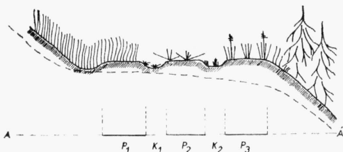
Obr. 5. — Schematický náčrt vegetace cesty na Z svahu Ještědu, schema A—Á: P 1 — přísvahový (vnitřní) pás vegetace, P 2 — střední pás, P 3 — svahový (vnější) pás, K 1 — vnitřní kolej, K 2 — vnější kolej. — Abb. 5. — Schematische Darstellung der Trittpflanzengesellschaften am W-Hange des Jeschken, Schnitt A—Á: P 1 — innere Vegetationsgürtel, P 2 — mittlere Vegetationsgürtel, P 3 — äussere Vegetationsgürtel, K 1 — innere Spur, K 2 — äussere Spur.
