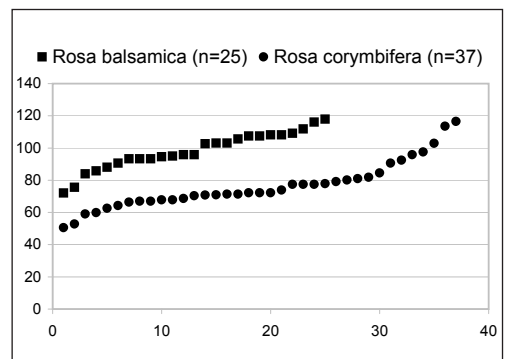
Abb. 6: Dicke von Blattfiedern der beiden Rosearten Rosa balsamica und R. corymbifera ; x-Achse: laufende Nr. der Blattfiedern (jedes Zeichen steht für 1 Exemplar); y-Achse: Dicke ( \mu ). – Thickness of leaflets of R. balsamica and R. corymbifera ; x-axis: serial number of the leaflets (each sign represents 1 leaflet); y-axis: thickness ( \mu ).
