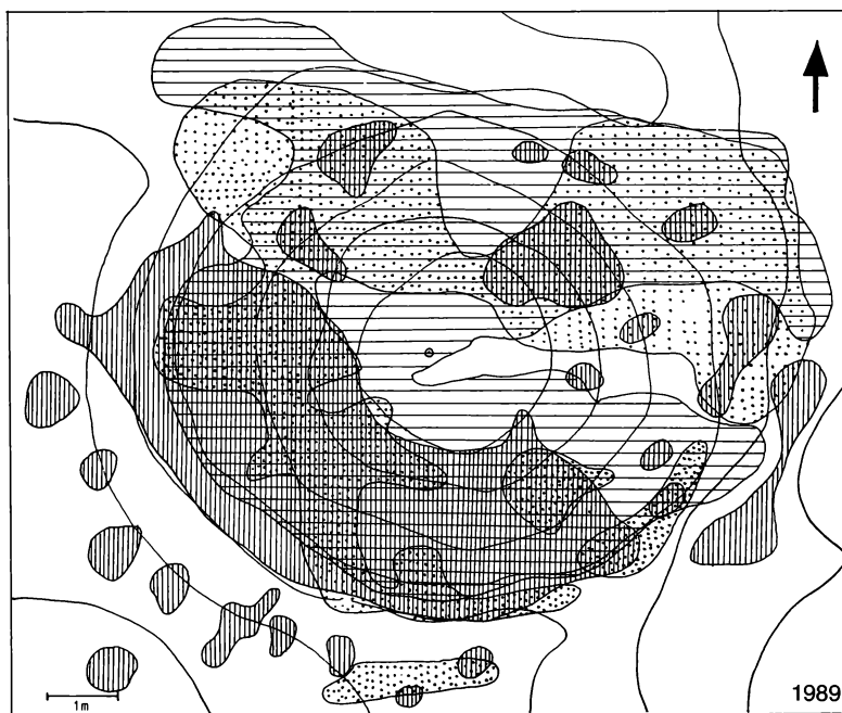
Abb. 4–7. Aufsichtsdiagramme der Galmeicharakterarten eines Pingentrichters aus den Jahren 1986–1989 (jeweils im Sept. erstellt)
