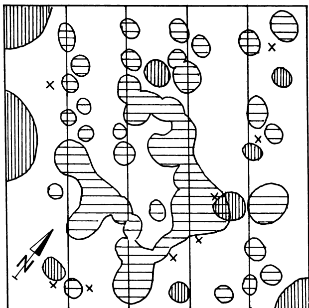
Abb. 8. Aufsichtsdiagramm eines Aussaatversuches (Sept. 1986) von Thlaspi calaminare (erstellt im Aug. 1989)
