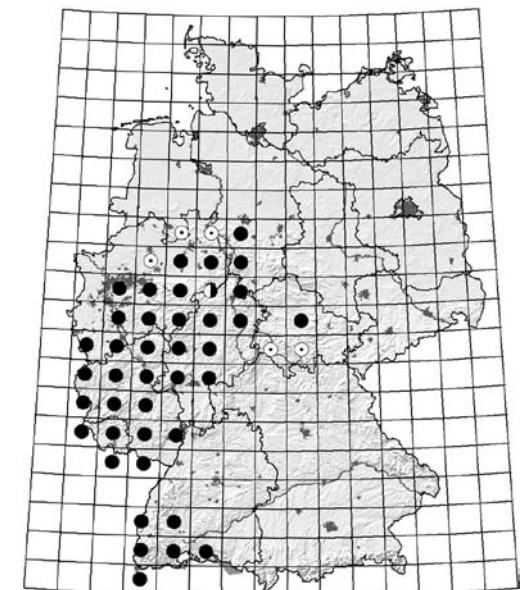
Abb. 3: Verbreitung von Pterostichus cristatus auf Basis der TK 100 Quadranten in Deutschland, Karte aus TRAUTNER et al. (im Druck). Kartenlegende: ○ Funde vor 1900, ⊙ Funde 1901-1950, ● Funde 1951-1980, ● Funde nach 1980.
