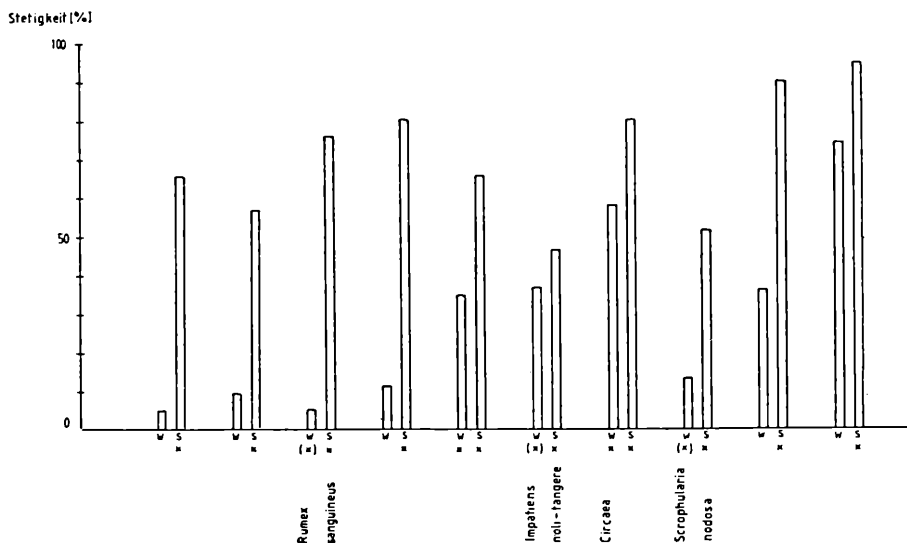
Abb. 12: Stetigkeit einiger Arten in Waldgesellschaften (w) und Saumgesellschaften (s) sowie deren Entwicklung x blüht und fruchtet (x) blüht und fruchtet teilweise
