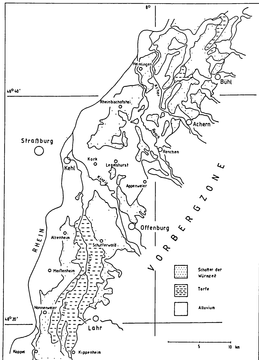
Abb. 2: Geologische Verhältnisse im Untersuchungsgebiet (nach: Geol. Übersichtskarte für S-W-Deutschland)
