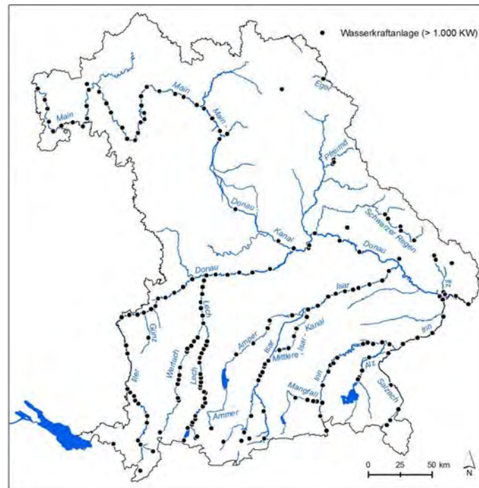
Abb. 12. Staustufen mit Wasserkraftanlagen zur Energiegewinnung (> 1000 kW) in Bayern (© Karte: Sabine Fischer Kartengrundlage Bayer. Vermessungsverwaltung und LfU).
