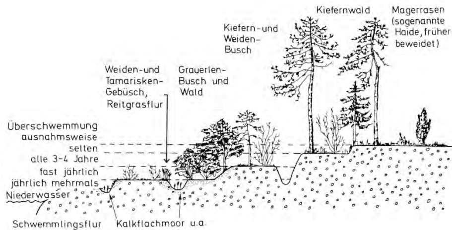
Abb. 2. Typische Zonierung der Aue im Ober- und Mittellauf eines alpinen Wildflusses vor Beginn der wasserbaulichen Maßnahmen (nach SEIBERT 1958 und MÜLLER 1991a aus ELLENBERG 1996).
