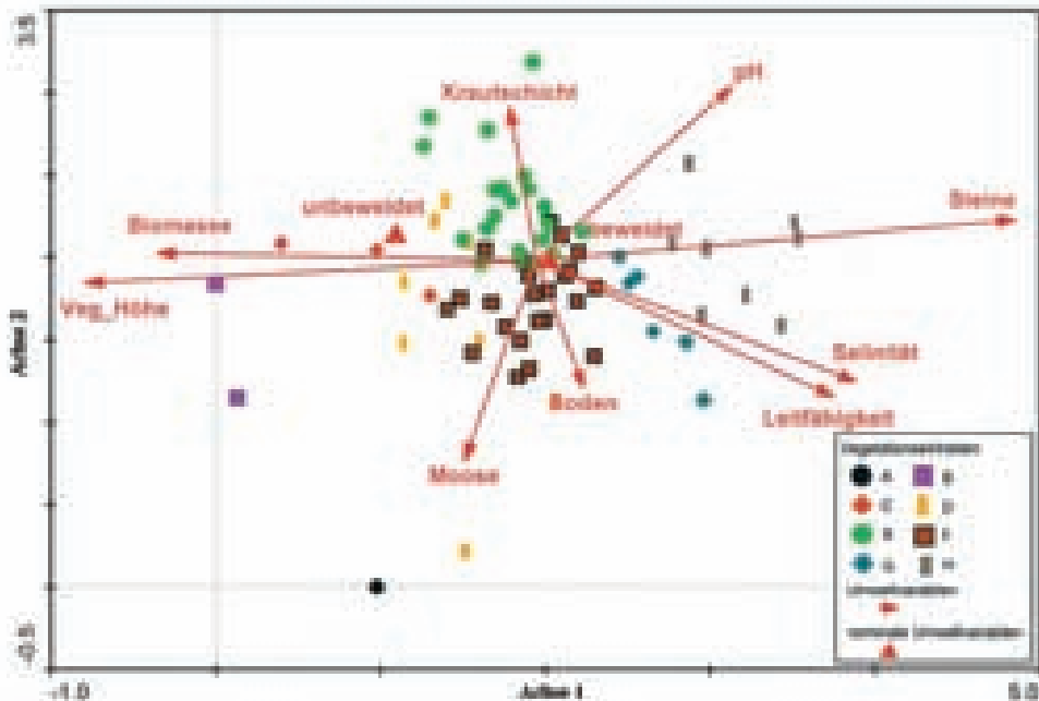
Abb. 6: Indirekte Gradientenanalyse (DCA) der Aufnahmen mit den erfassten Umweltvariablen. Die Aufnahmen wurden entsprechend der in TWINSPLAN ermittelten Vegetationseinheiten den Gruppen A–H zugeordnet. Eigenvalues: Achse 1, 0,30; Achse 2, 0,18. Abkürzungen der Umweltvariablen: beweidet: beweidete Aufnahmeflächen; Biomasse: Trockenbiomasse der Probestellen; Krautschicht: Deckung der Krautschicht; Leitfähigkeit: Leitfähigkeit der Bodenproben; Moose: Deckung Moosschicht; pH: Reaktion Bodenproben; Salinität: Salinität Bodenproben; Steine: Deckung Steine; unbeweidet: unbeweidete Aufnahmeflächen; Veg_Höhe: mittlere Höhe der Vegetation.
