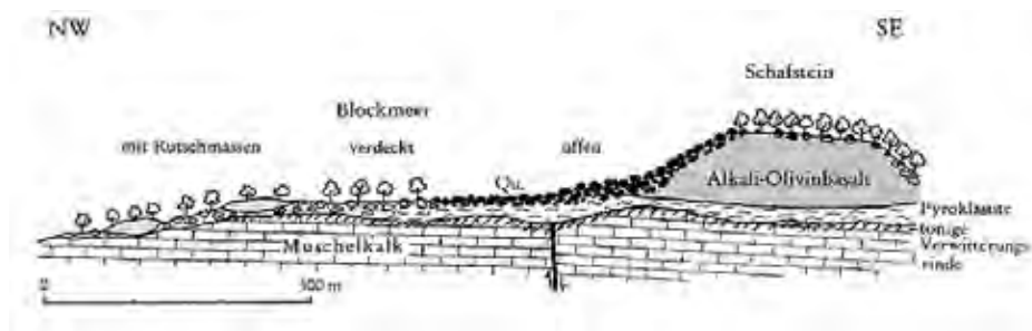
Abb. 3.4/9: Geologischer Längsschnitt durch das Basaltblockmeer am Schafstein (EHRENBERG et al. (1994) nach MENSCHING (1960), umgezeichnet und ergänzt von LAEMMLER).
