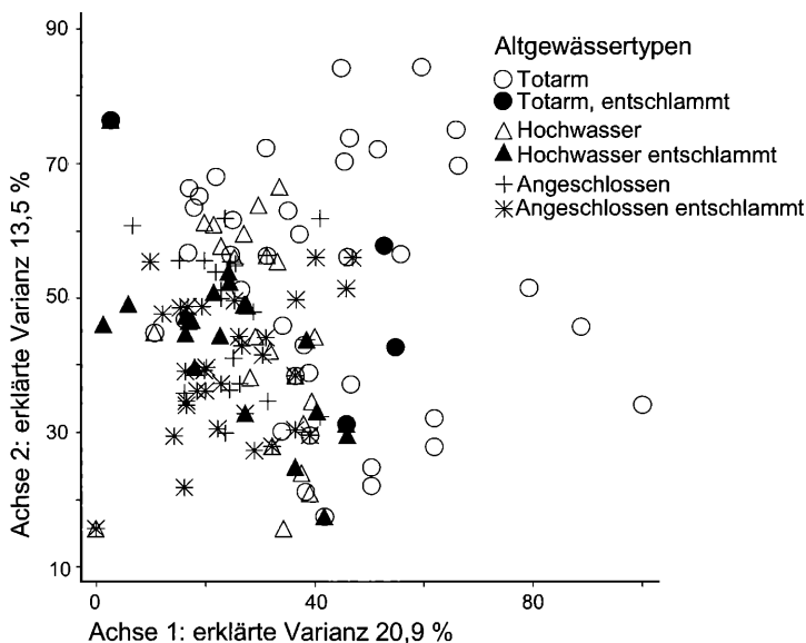
Abbildung 3: Ordination der Vegetationsaufnahmen der aquatischen Aufnahmequadrante durch eine DCA. Die Signaturen kennzeichnen den Fließgewässereinfluss und den Einfluss der Entlandungsmaßnahmen.
