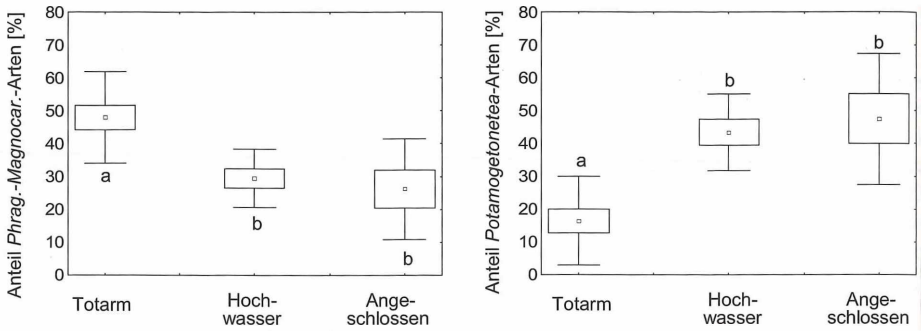
Abbildung 4: Einfluss des Fließgewässers auf die Anteile der Phragmiti-Magnocaricetea -Arten (links) und der Potamogetonetea -Arten (rechts) an der Gesamtartenzahl in den aquatischen Altarmabschnitten. Die Box-Plots zeigen Mittelwert (□), Standardfehler und Standardabweichung. Unterschiedliche Buchstaben zeigen statistisch signifikante Unterschiede ( p < 0,05 ).
