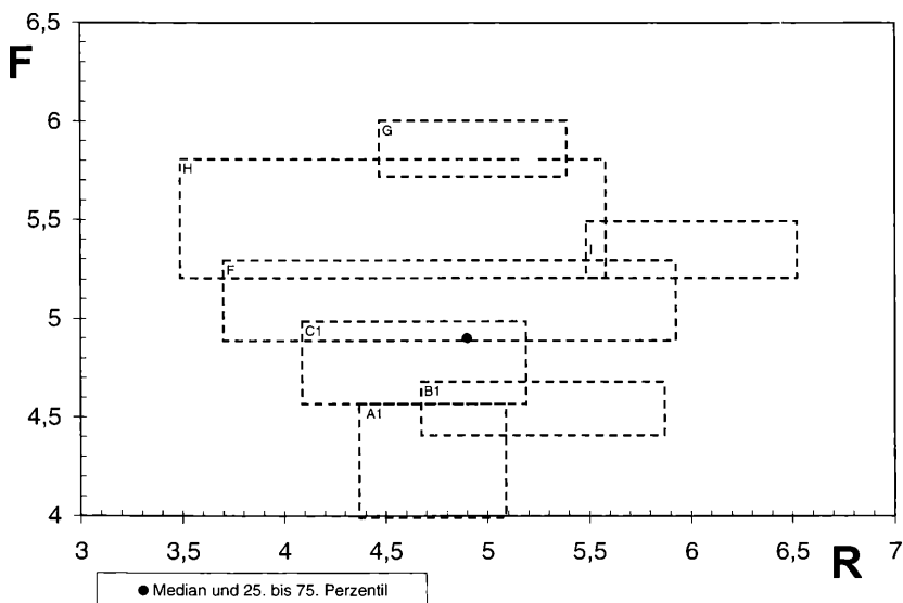
Abb. 6: Reaktionszahl-Feuchte-Ökogramm - Fragmentgesellschaften.
