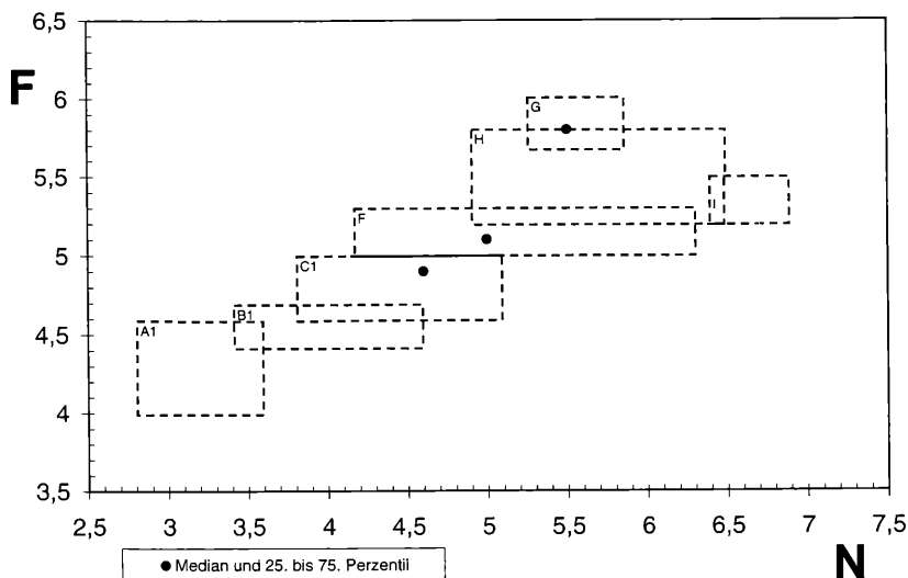
Abb. 5: Nährstoff-Feuchte-Ökogramm - Fragmentgesellschaften.
