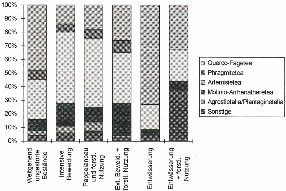
Abb. 3: Änderung der Deckungsanteile von Arten verschiedener soziologischer Gruppen in der Feldschicht von Hartholzwäldern der Mittel- und Oberelbe bei unterschiedlicher Störung (kalkuliert auf der Basis von insgesamt 30 Vegetationsaufnahmen)
