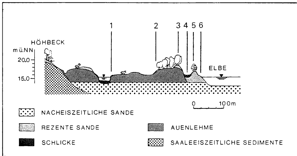
Abb. 1: Schematischer Querschnitt durch die Elbaue bei Pevesdorf. Erkennbar sind Geomorphologie und räumliche Anordnung wichtiger Bodentypen im Gebiet; 1: Auennaßgley, 2: Allochthone Vega, 3: Autochthone Vega, 4: Auenanmoorgley, 5: Paternia, 6: Rambla (aus MEYER & MIEHLICH 1983, etw. verändert).
