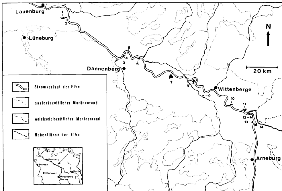
Abb. 2: Lage und Bezeichnung der untersuchten Hartholzauen im Gebiet der Unteren Mittelbe; 1: Achterholz, 2: Vitico, 3: Penkefitz-Jasebeck, 4: Jasebeck, 5: Jasebeck (Außendeichsflächen), 6: Wulfsahl (Außendeichsflächen), 7: Elbholz, 8: Garbe, 9: Wahrenberg, 10: Rühstätt, 11: Quizöbel, 12: Werben, 13: Röbel, 14: Havelberg.
