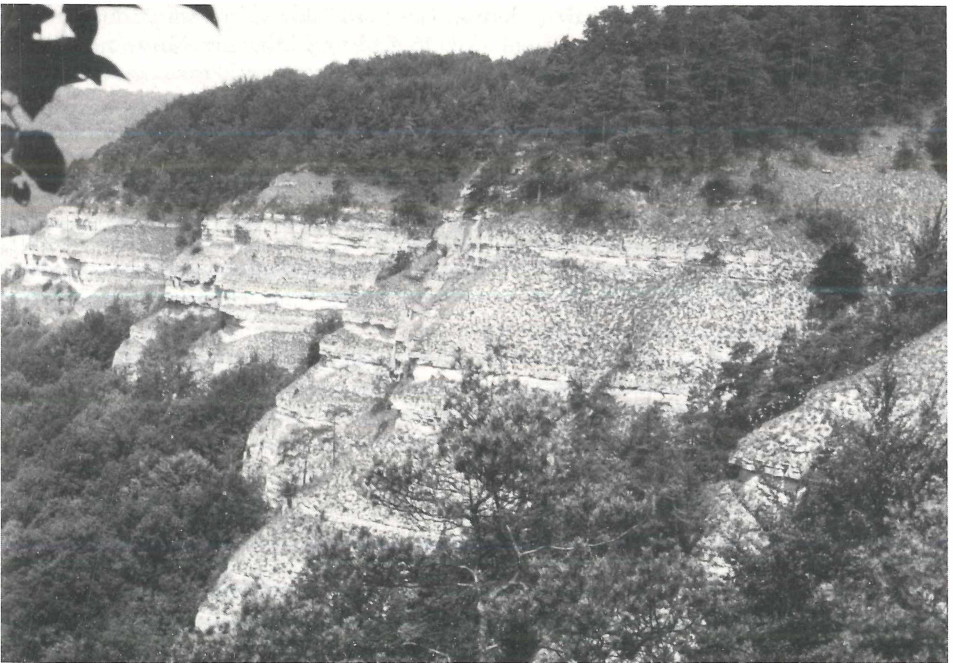
Abb. 3: Nordmannsteine bei Ebenau; auf den als Werra-Prallhang entstandenen Muschelkalkhängen stößt der Wald an eine natürliche Trockengrenze. Die waldfreien Partien werden von Blaugrashalden ( Teucrio-Seslerietum ) besiedelt
