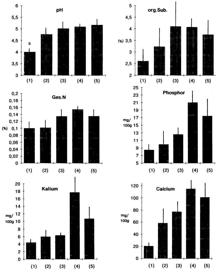
Abb. 1: Pedologische Kennwerte der soziologischen Einheiten
