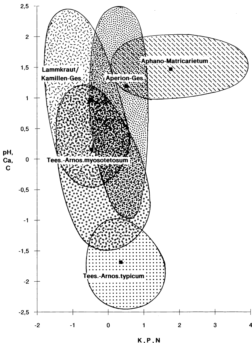
Abb. 2: Diskriminanzanalyse der Bodenkennwerte der soziologischen Einheiten.
