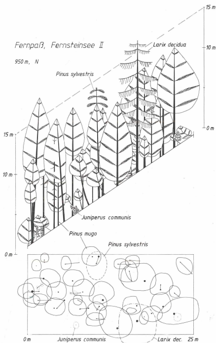
Abb. 7: Grund-/Aufriß eines Lycopodium annotini -Mugetum prenanthetosum : Seehöhe: 950 m, Exposition: N; Alter: ca. 210 Jahre, Vorrat: 150 fm/ha (Spirke: 121 fm/ha, Lärche: 20 fm/ha, Föhre: 9 fm/ha).
