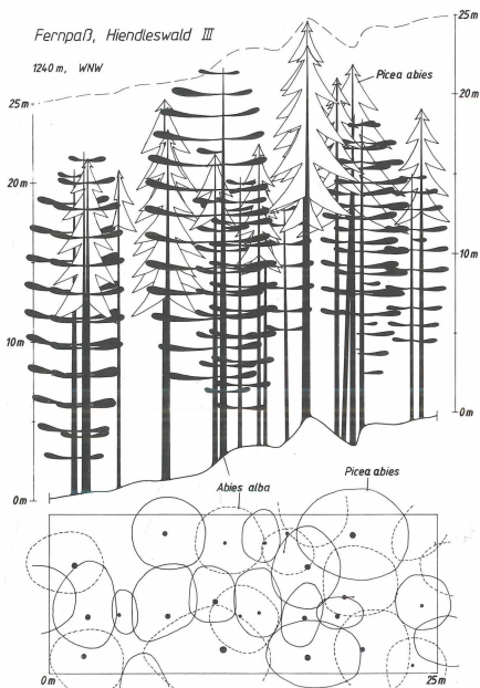
Abb. 1: Grund-/Aufriss eines Adenostylo glabrae-Abietetum : Seehöhe: 1240 m, Exposition: WNW; Alter: ca. 140 Jahre, Vorrat: 535 fm/ha (Fichte: 322 fm/ha, Tanne: 213 fm/ha).
