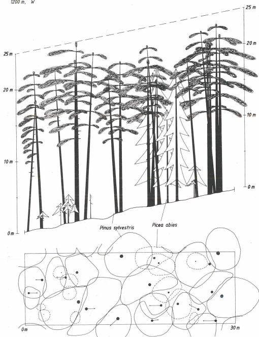
Abb 3: Grund-/Aufriß eines Erico-Pinetum sylvestris bylcomietosum , Melampyrum sylvaticum -Variante: Seehöhe: 1200 m, Exposition: W; Alter: ca. 140 Jahre (Fichten bis ca. 190 Jahre), Vorrat: 625 fm/ha (Föhre: 570 fm/ha, Fichte: 55 fm/ha).
