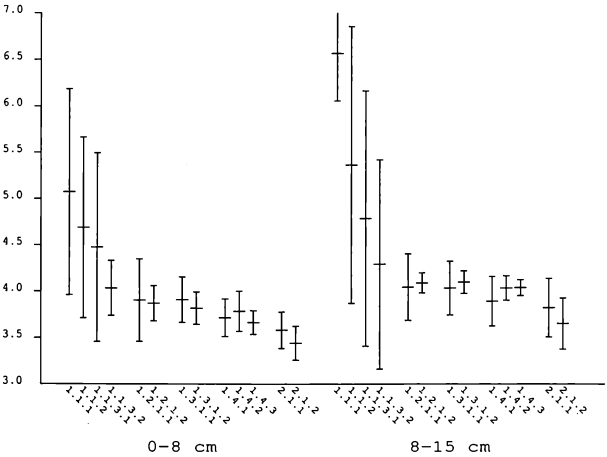
Abb. 5: pH-Werte (KCl) der verschiedenen Vegetationseinheiten in zwei Bodentiefen (Mittelwert und Streuung).
