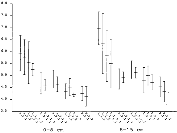
Abb. 4: pH-Werte (H 2 O) der verschiedenen Vegetationseinheiten in zwei Bodentiefen (Mittelwert und Streuung).
