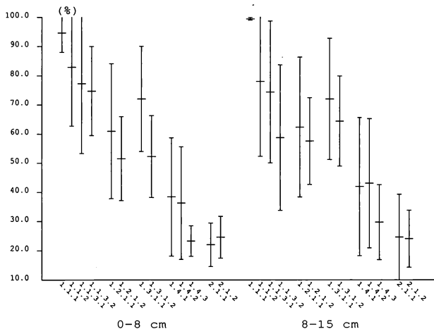
Abb. 6: Basensättigung der verschiedenen Vegetationseinheiten in zwei Bodentiefen (Mittelwert und Streuung).
