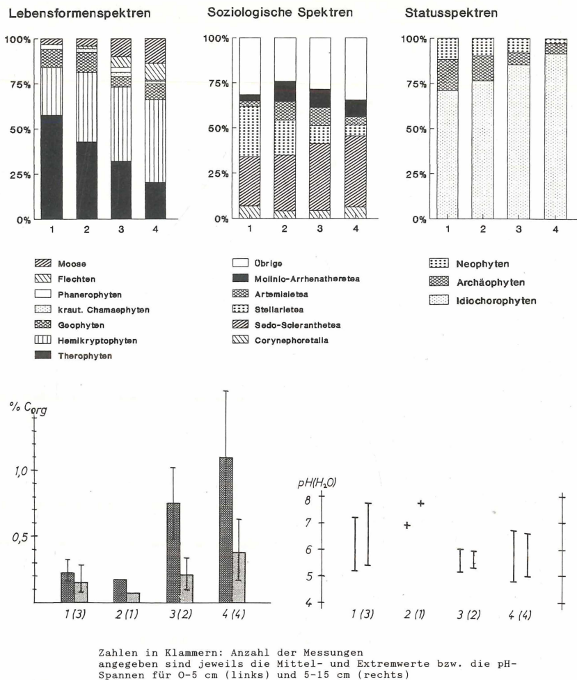
Abb. 7: Spektren (oben) und bodenchemische Standortsverhältnisse (unten) der Sukzessionsphasen auf nährstoffreichen Moränensanden.
