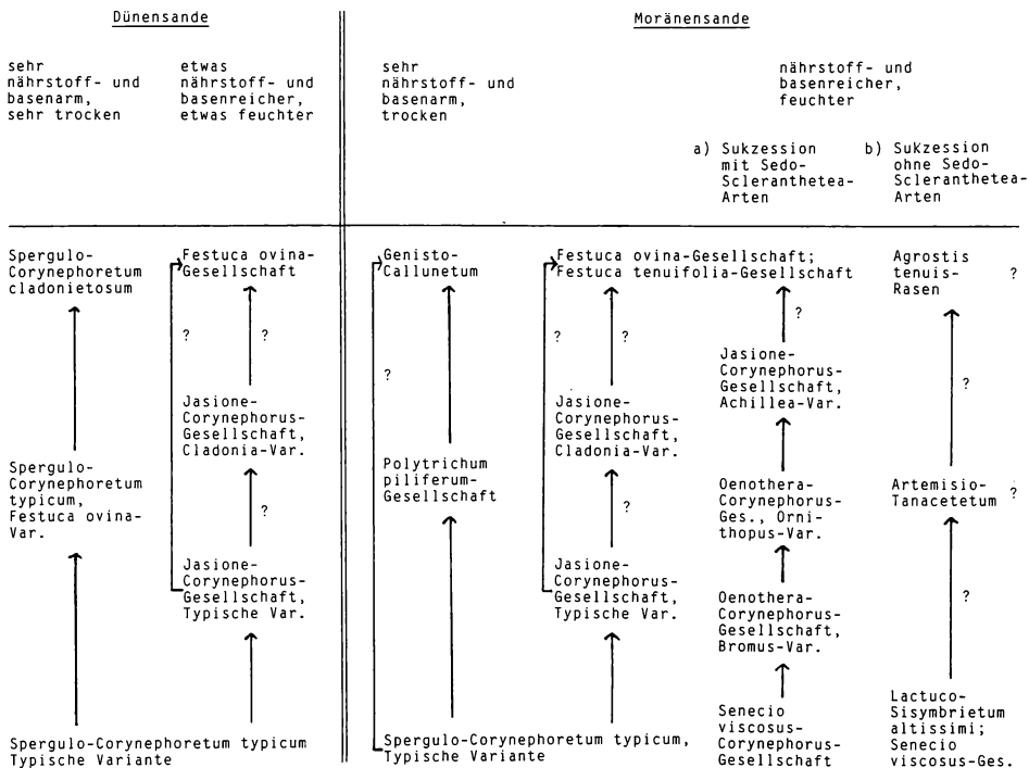
Abb. 2: Sukzessionsschema der Besiedlung von Sand-Rohböden im Untersuchungsgebiet.
