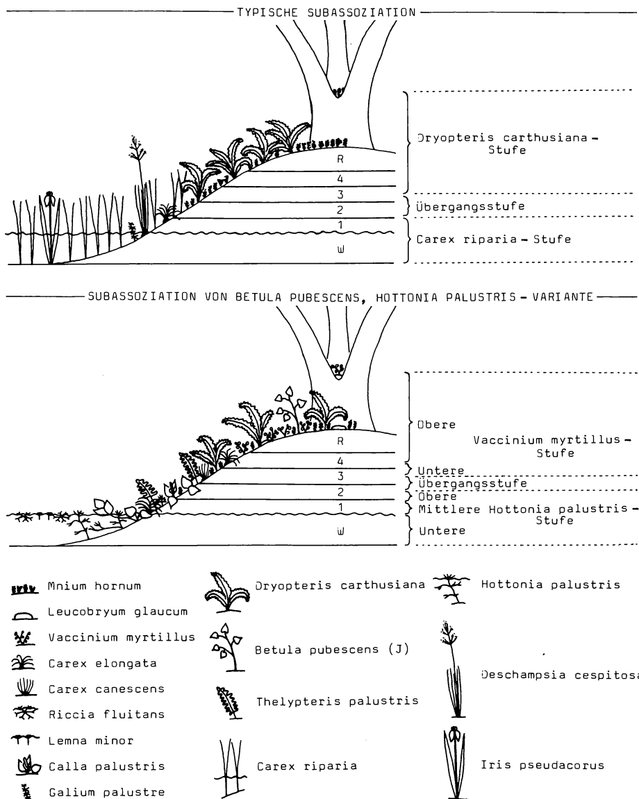
Abb. 5: Vegetationsabstufung der Bulten-Schlenken-Komplexe in Erlenbruchwäldern des Hannoverschen Wendlands.
