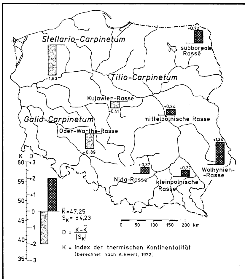
Abb. 2: Koinzidenz der regional-syntaxonomischen Gliederung der Eichen-Hainbuchenwälder Polens mit dem Kontinentalitäts-Gefälle des Klimas.
