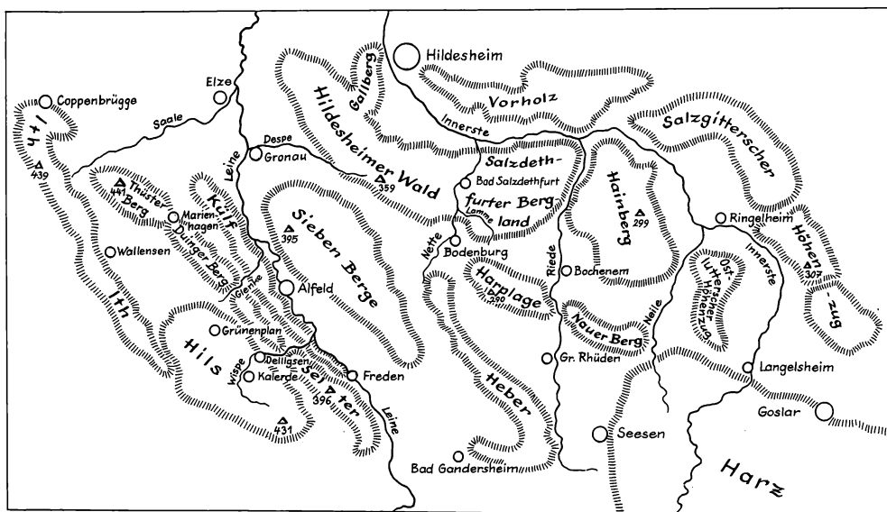
Mittelleine - Innerste-Bergland
