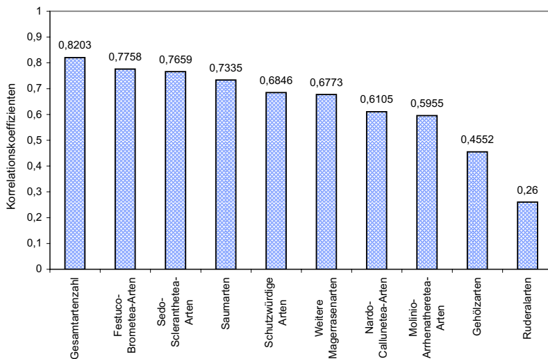
Abb. 13: Vergleich der Korrelationskoeffizienten (Spearman-Rang-Test) der typischen Artengruppen im Bezug zur Flächengröße der Porphyrkuppen (aus PARTZSCH & MAHN 1998).
