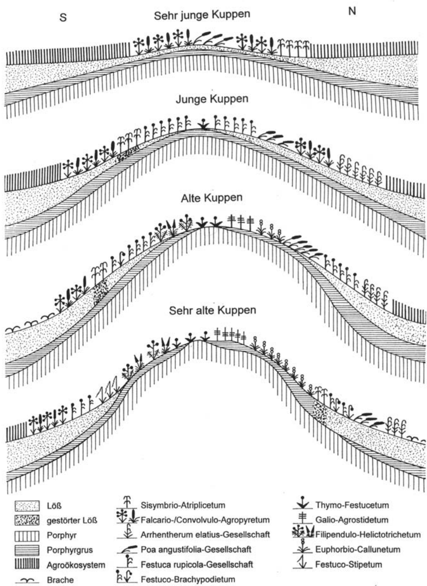
Abb. 17: Schematische Darstellung des Vegetationsmosaiks auf den Porphyrykuppen in Abhängigkeit von der Genese der Standorte (aus PARTZSCH 2001). Fig. 17: Vegetation mosaics of the porphyry outcrops in dependence on the genesis of the location (from PARTZSCH 2001).
