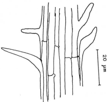
Stiel
