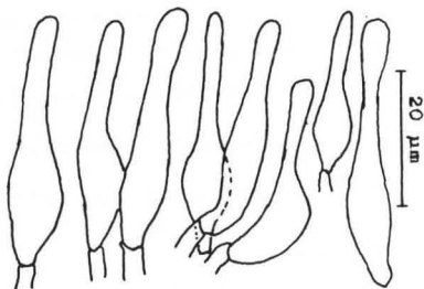
Cheilozytisten
