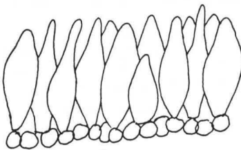
Huthaut
