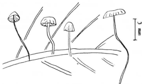
Fruchtkörper
