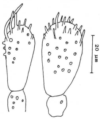
Huthaut
