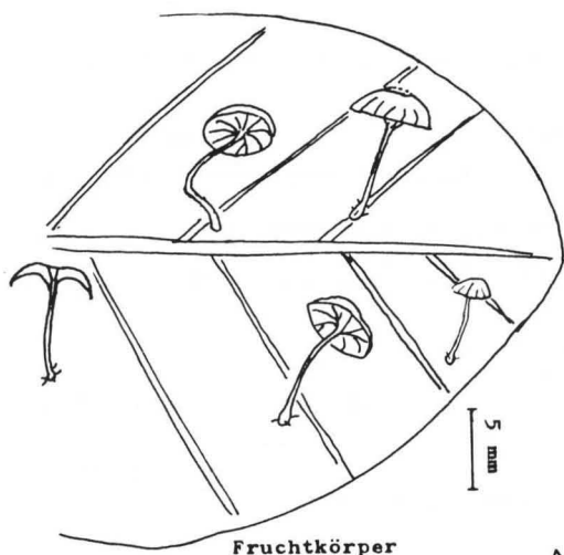
Fruchtkörper
