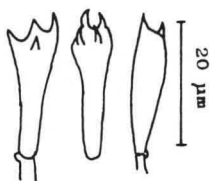
Basidien
