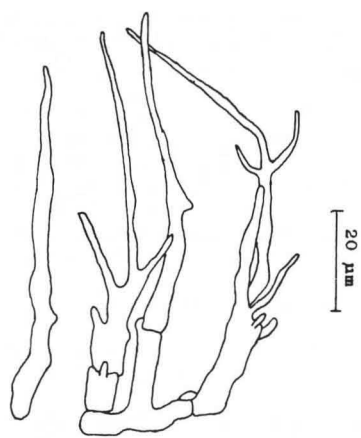
Kaulozystiden
