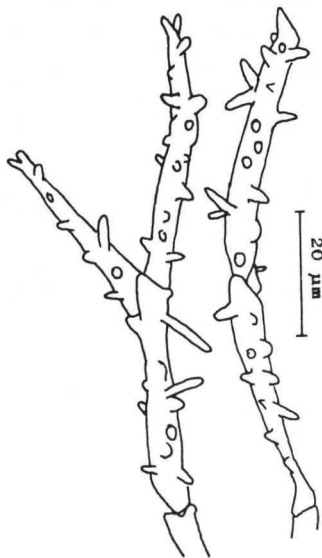
Huthaut
