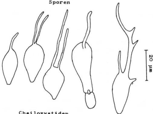
Cheilozystiden
