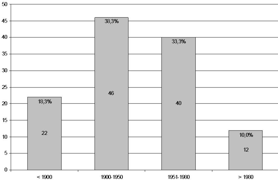
Abb. 2: Häufigkeitsverteilung der in Hessen ausgestorbenen Pflanzenarten, aufgeschlüsselt nach Aussterbezeiträumen mit Angabe der absoluten Zahl und des prozentualen Anteils.
