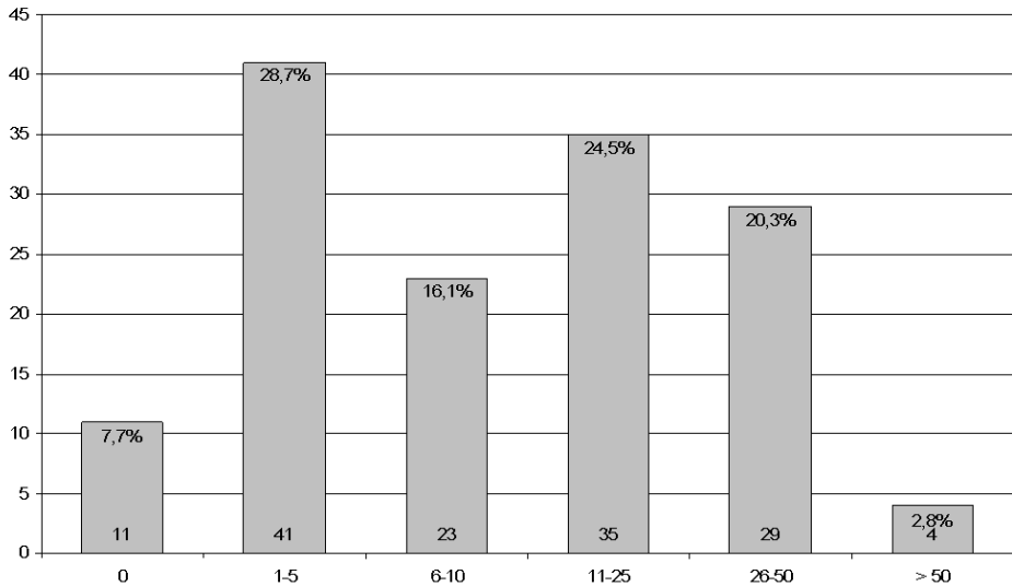
Abb. 1: Häufigkeitsverteilung der aus Hessen stammenden Herbarbelege zu den als ausgestorben oder verschollenen geltenden Arten mit Angabe der absoluten Zahl und des prozentualen Anteils.
