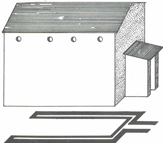
RÖMISCHER TROCKENOFEN
