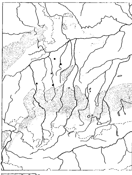
Tettigonia cantans
