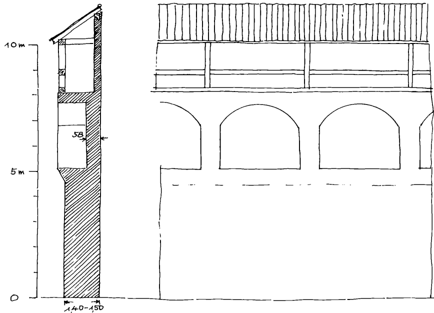
Stadtmauer an der Schlossermauer (in Wohnhäuser eingebaut) Backsteine 7,5-8cm/37/18
