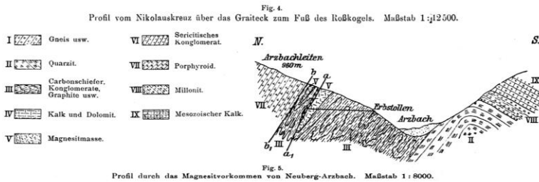
Abb. 4: Profile durch die Magnesitlagerstätten bei Veitsch und Neuberg-Arbach, Steiermark, aus Redlich 1913
