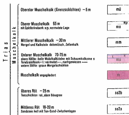
Abb. 3: Geologie des Naturschutzgebietes und seiner Umgebung; aus der Geologischen Karte 1:25 000 Nr. 5734 Wallenfels
