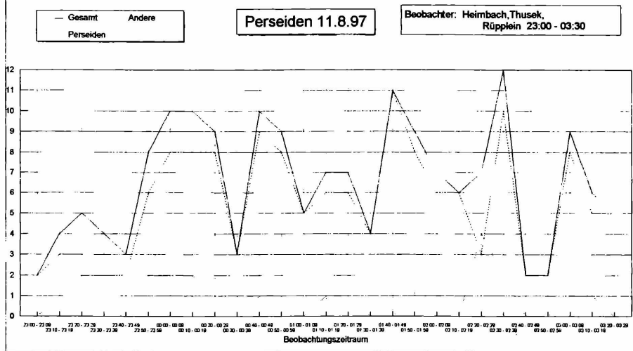
Abb. 1: Häufigkeitsverteilung der beobachteten Perseidenfälle im Bezugszeitraum 11.-12.08.1997, 23.00-3.30 Uhr
