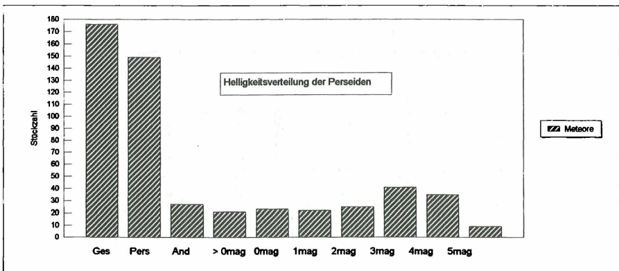
Abb. 2: Verteilung der Helligkeitsklassen der beobachteten Perseidenfälle im vorgenannten Zeitraum
