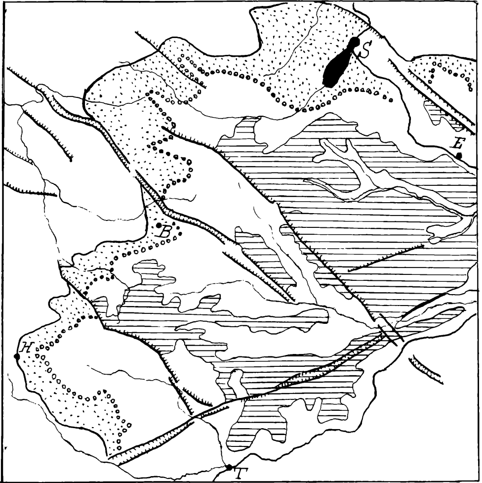
Abb. 12 Der Einfluß des Fildergrabens auf den Stufenrandverlauf. Horizontal schraff. Lias-Decke erhalten. Kreislinie: Stubensandsteinrand. Durchgehende Linie: Gipskeuperrand. S Stuttgart, B Böblingen, E Esslingen, H Hechingen, T Tübingen.
