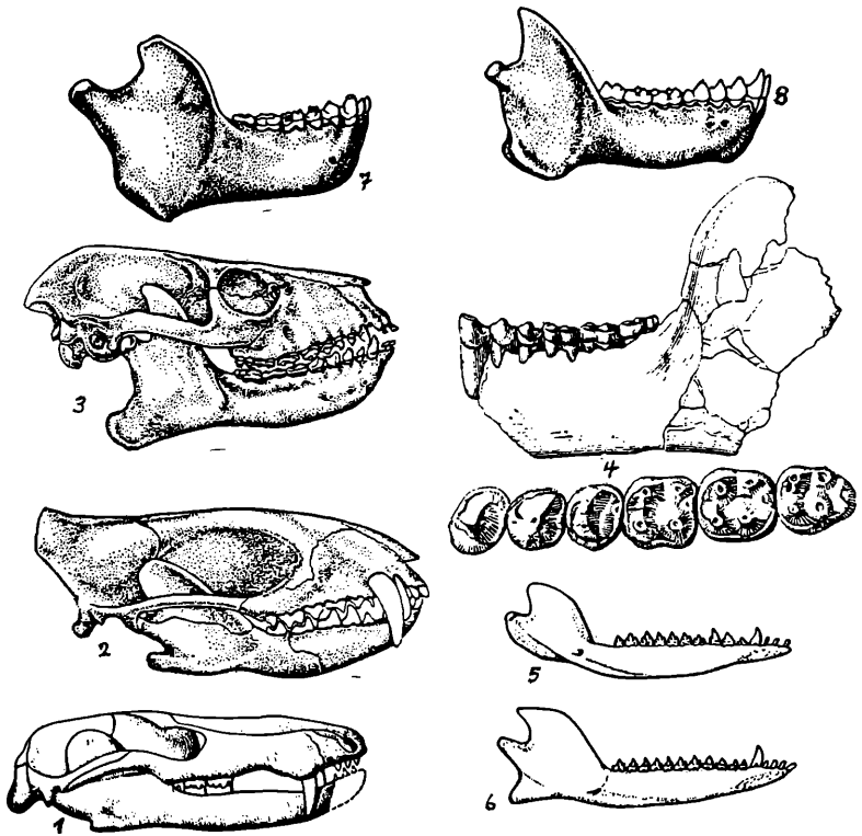
Abb. 8 1 - 3 Schädel aus der ältesten Evolution der Säugetiere, in aufsteigender Folge.
