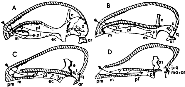
Abb. 15 Oben Proportionen der Gliedmassen bei Höheren Primaten. a Orang-Utan, b Schimpanse, c Gorilla, d Mensch. Aus KUHN-SCHNYDER
