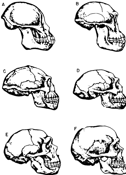
Abb. 17 Schädel höherer Primaten.
