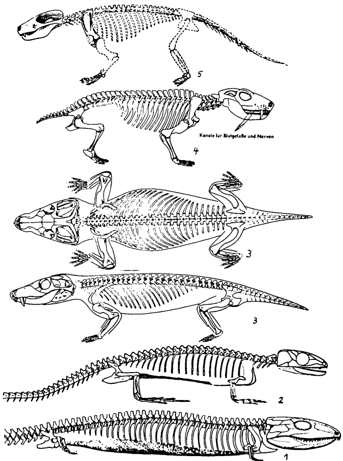
Abb. 9 Skelette primitiver Tetrapoden in aufsteigender Reihenfolge.
