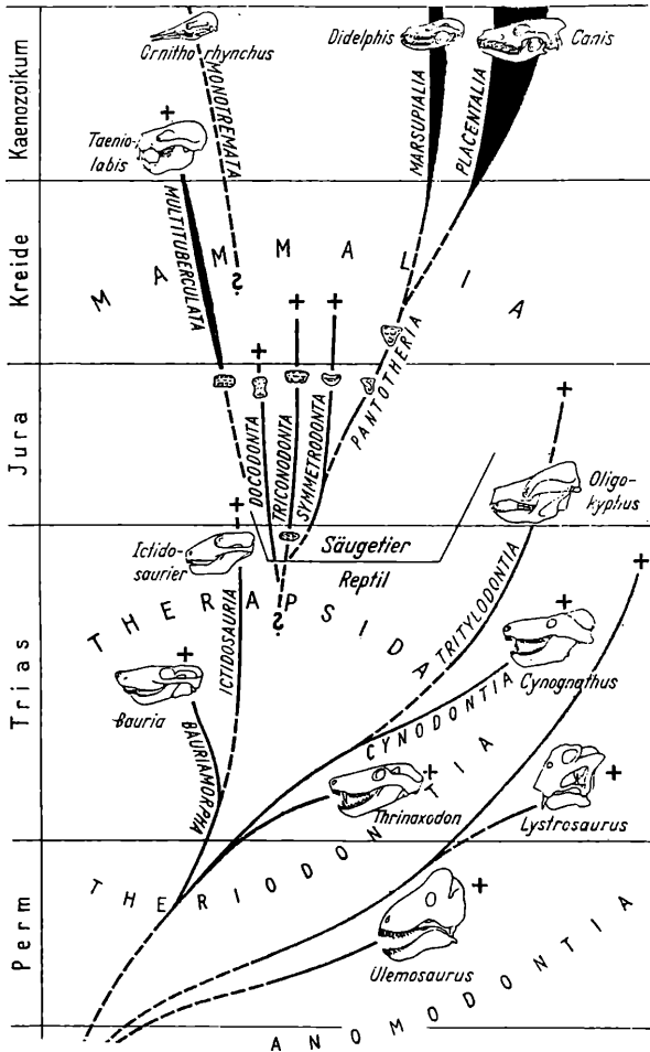
Abb. 13b Die stammesgeschichtlichen Beziehungen der Therapsida zu den Säugetieren, Angleichung verschiedener Reptilllinien an die Säugetiere. Nach E. THENIUS 1960
