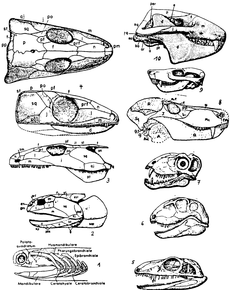
Abb. 7 Schädel von 9 Fischen und Tetrapoden, angeordnet in der Reihe aufsteigender Entwicklung zu den Säugetieren hin (letzte sind nicht berücksichtigt).
