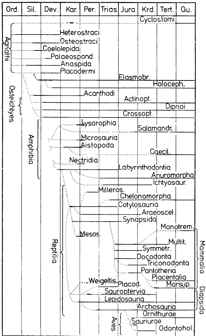
Abb. 1 Stammbaum der Wirbeltiere, es sind alle Klassen und Unterklassen berücksichtigt, nur die Placodermen (mit 9 Ordnungen bzw. Unterklassen) wurden als Einheit dargestellt. Original.
