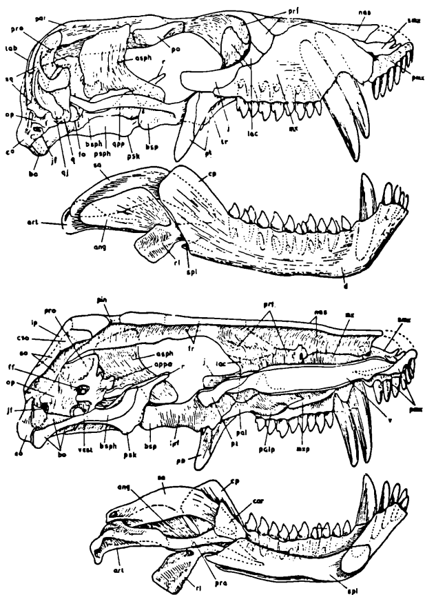
Abb. 11 Schädelbau eines Bauriamorphen, in der Wand der Gehirnkapsel ein großes Epipterygoid (Alisphenoid der Säugetiere); Unterkiefer von der Innen- und Außenseite. Nach BRINK.
