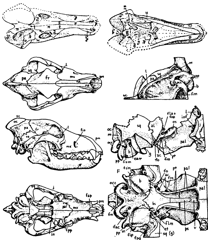
Abb. 12 Oben Schädel des Therocephalen Alopecognathus , nach BOONSTRA
