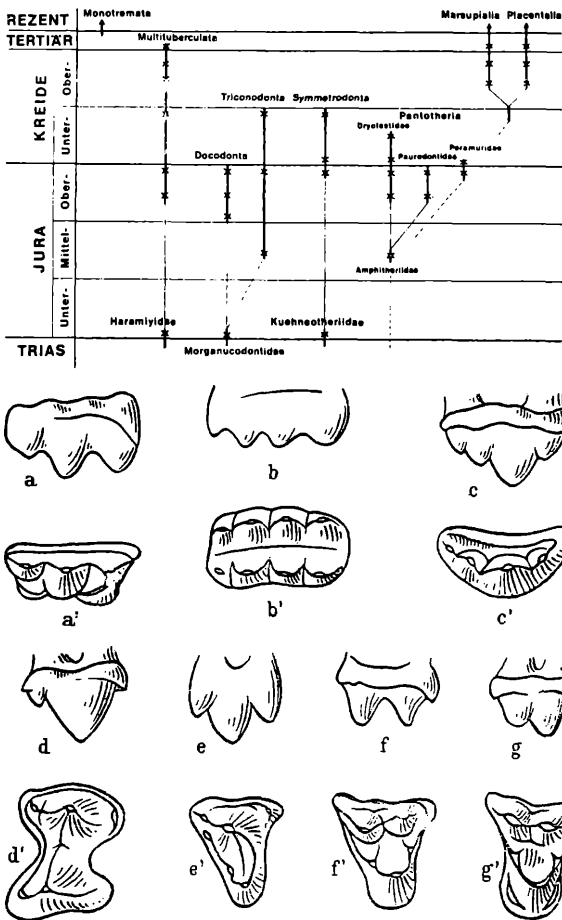
Abb. 14 Oben Stammbaum der Unterklassen der Säugetiere, dicke Linien bedeuten die nachgewiesene Lebensdauer, dünne Linie gesicherte Beziehung, gestrichelt wahrscheinliche Beziehung, x Funde. Nach B. KREBS 1975
