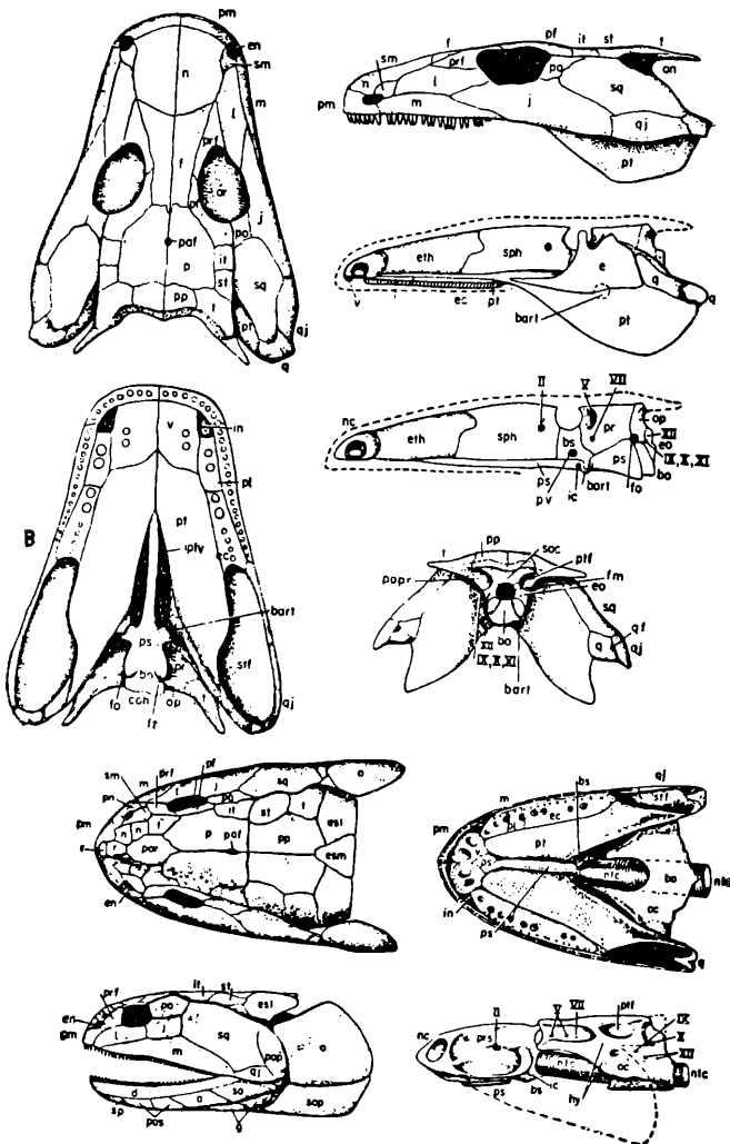
Abb. 5 Oben Schädel des karbonischen Anthracosauriers Palaeogyrinus Unten Schädel des devonischen Crossopterygiers Eusthenopteron . Schädel in 4 Ansichten und die Neuralcranien. Nach A.S. ROMER
