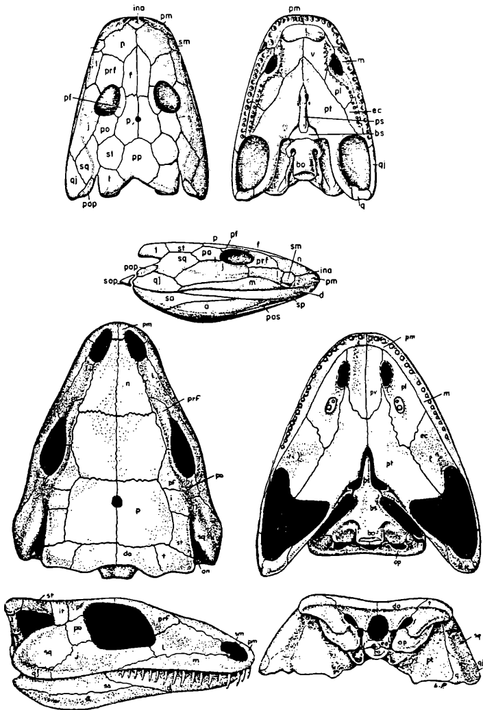
Abb. 6 Oben Schädel des oberdevonischen Labyrinthodonten Ichthyostega in 3 Ansichten. Unten Schädel des altpermischen Labyrinthodonten Seymouria , in 4 Ansichten. Nach A.S. ROMER
