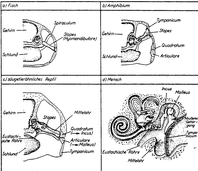
Abb. 13a Das Gehörorgan in der Wirbeltierreihe. Nach A.S. ROMER, aus A.H. MÜLLER.
