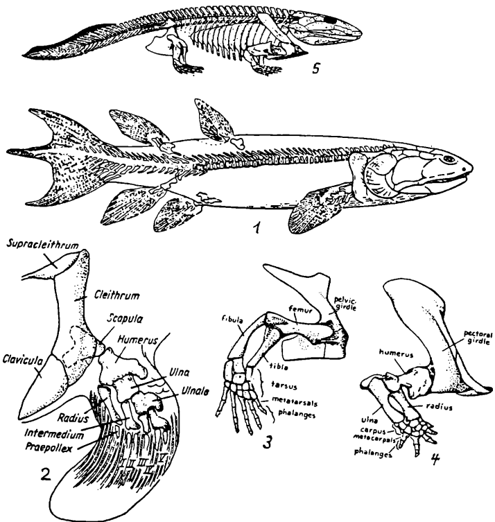
Abb. 4 Das Verhältnis der Crossopterygier (Eusthenopteron) zu den Amphibien (Ichthyostega).
