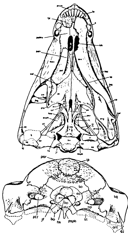
Abb. 10 Aneugomphius , ein Therocephale, Gaumen und Hinterhaupt, letzteres fast 12 cm breit. Nach BRINK.
