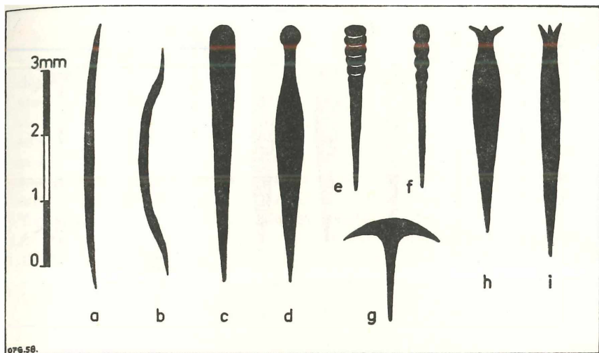
Abb. 1 Isolierte Spicula aus Weißjura \gamma von Würgau (Oberfranken); a-b = Amphiox, c = Styl, d = Tylostyl, e-f = Criccostyl, g = Ancriox, h-i = Prostylotriaen; aufbewahrt im Geol.-Paläont. Inst. TH. Stuttgart.
